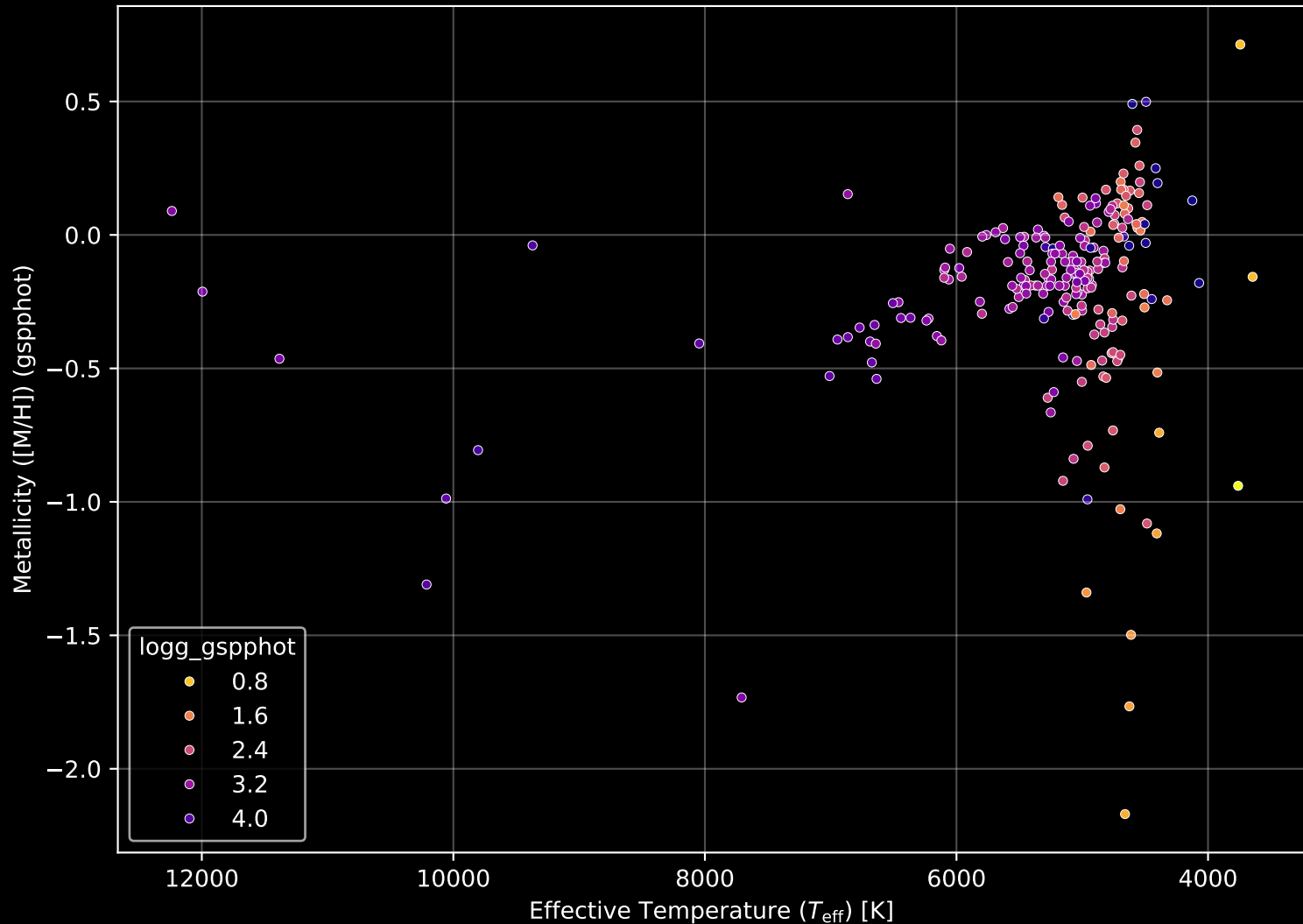
APOGEE DR17 Field: [NGC7789_btx] Stellar Population Parameters (n= 230)
